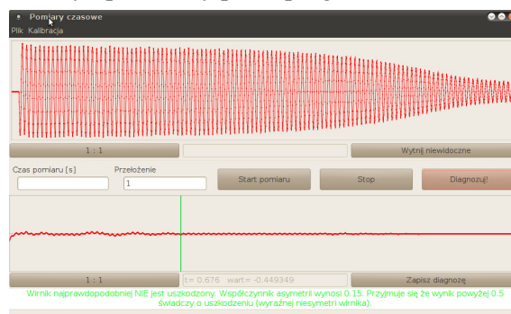
Rys. 1. Okno programu z zaimplementowaną procedurą diagnostyczną – wynik dla zdrowego silnika
